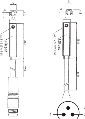
M 8 - Stecker
