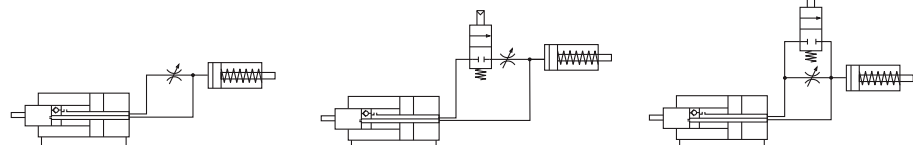
① Geschwindigkeitsregelung ② STOP-Ventil (Blockierventil) ③ SKIP-Ventil (Sprungventil)
