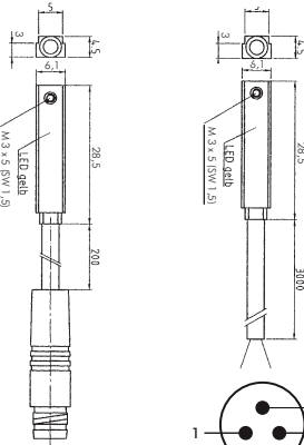
M 8 - Stecker
