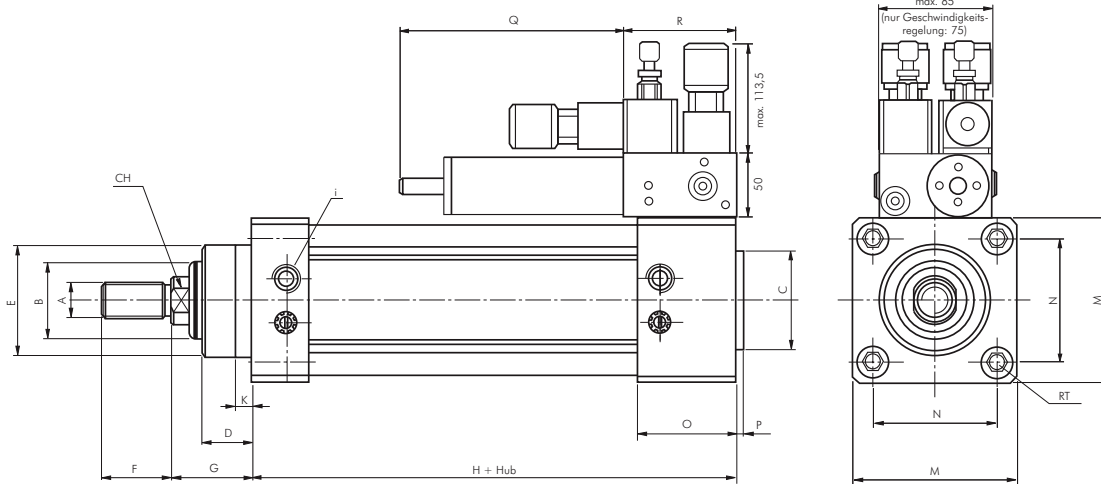
Maßtabelle für Ölbremsszylinder
