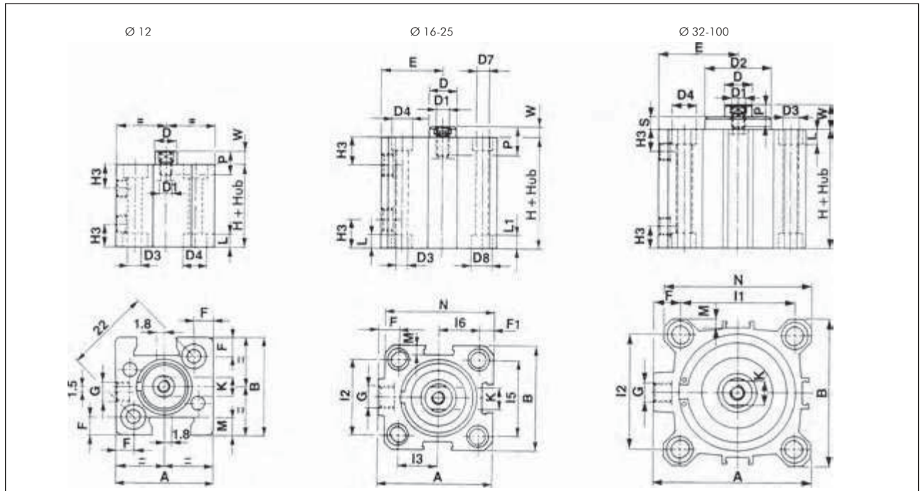
Maßtabelle für Kurzhubzylinder (doppeltwirkend) Typ ND/NDM
